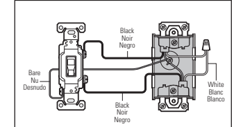
Identifier le câblage existant (ce commutateur sera unipolaire)
