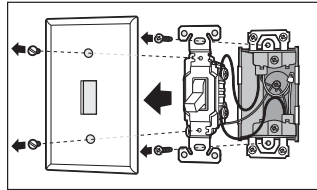
Quitar la placa de pared existente y tirar del interruptor
