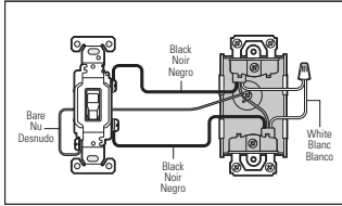
Identificar el cableado existente (este interruptor será unipolar)
