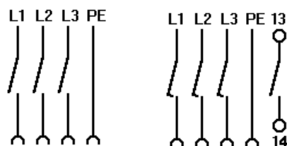
GHG 514, 4 pôles 50/60 Hz
