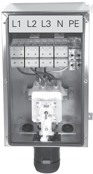
Terminals PE
