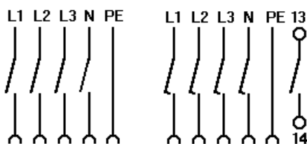
GHG 514, 5 pôles 50/60 Hz
