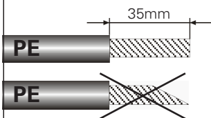
Terminals PE
