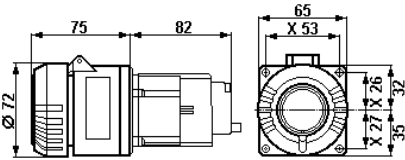
Flange socket 4/5-pol./ + PE
