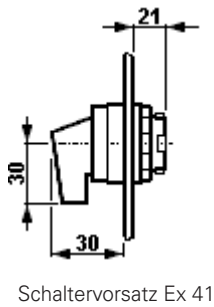
Schaltvorsatz Ex 41
