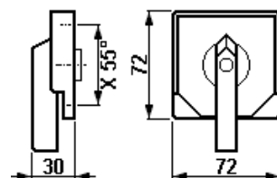
Schaltervorsatz Ex 28 / Ex 29
