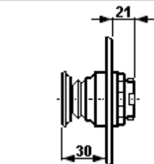
Schlagtastervorsatz "NOT-AUS"
