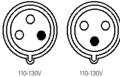
GHG 511, 2-pol.+PE
