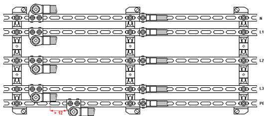
Fig. 3 Système de jeu de barres- raccordement vertical
