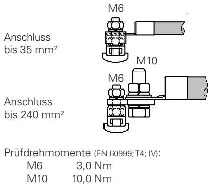
Bild 1 Anschlussbilder
