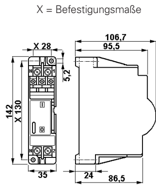
Komponentengröße 0 Module size 0 Tailles d' modules 0
