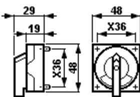
Schaltervorsatz Ex 23
