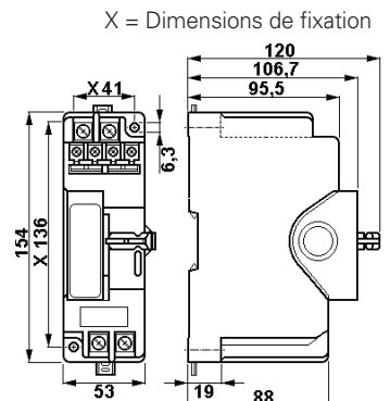
Komponentengröße 2 Module size 2 Tailles d' modules 2
