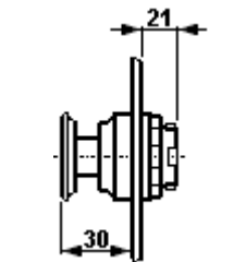
Schlagtastervorsatz X = Befestigungsmaße
