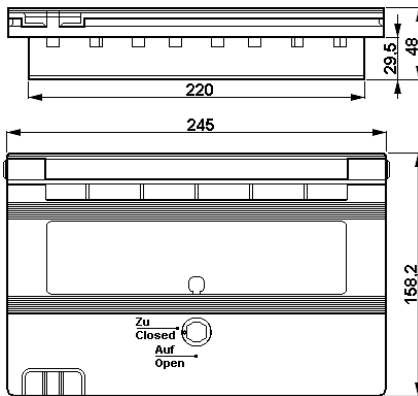
Klappe Größe 2 für GHG 61
