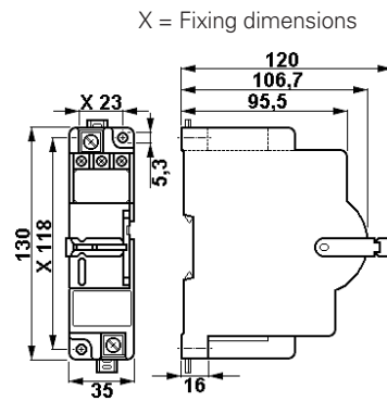
Komponentengröße 1 Module size 1 Tailles d' modules 1
