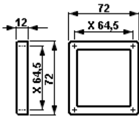
Messinstrumentenvorsatz M 72
