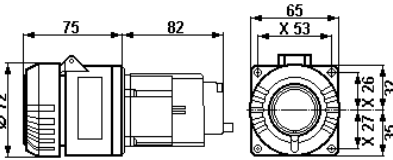
Flanschsteckdose 4/5-pol. + PE
