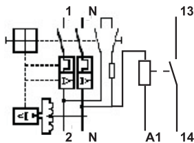
Bild 1.5.2 Anschlussbild FI- Schutzschalter mit Leistungsschalter und Interface Relais R1561
