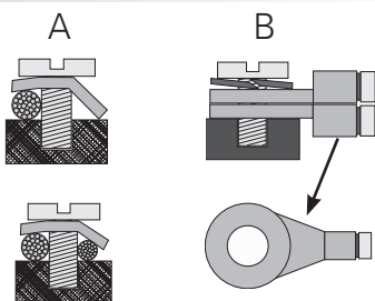
Bild 1.3.a Anschluss Haupt-; Hilfs-/Signalkontakte
