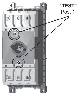
Bild 1.5 FI Prüftaste
