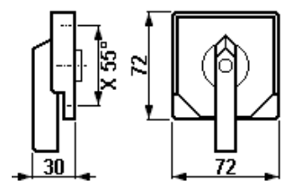
Switch actuator Ex 28 / Ex 29
