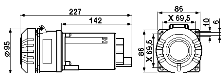
Prise à bride 3-pôl. + PE
