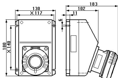
Prise murale sans interrupteur à 5 pôles
