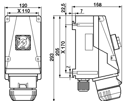
Wandsteckdose mit Schalter 5-polig
