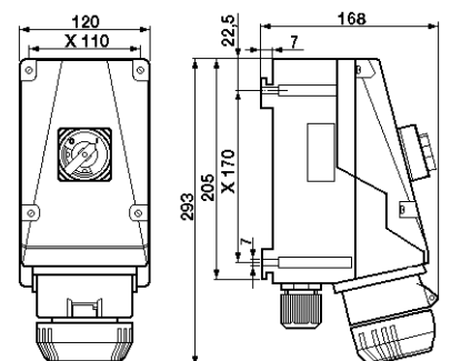
Prise murale avec interrupteur à 5 pôles
