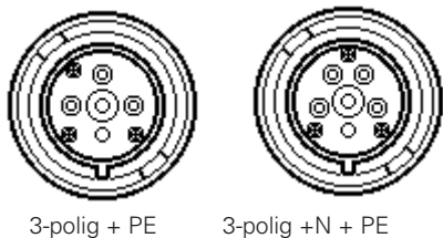
3-polig + PE 3-polig +N + PE
