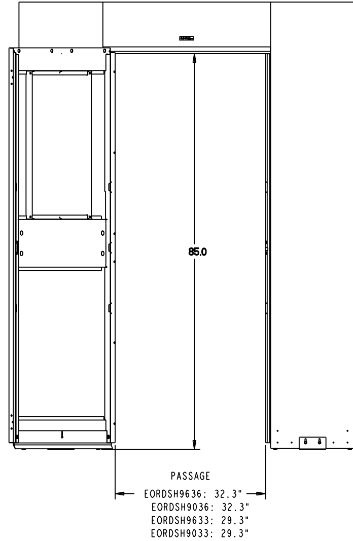
DOOR OPEN
