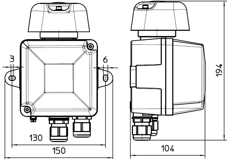
Maßbild / Dimensions
