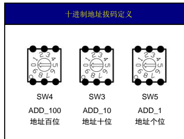
图 2.3.5.1. 拨码开关
