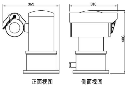
图 1.4.1.1 产品外形尺寸
