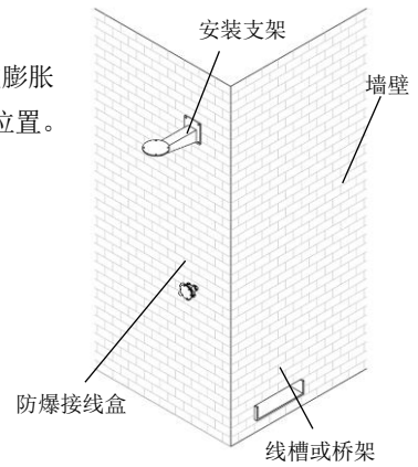
图 2.4.1.1 安装支架和接线盒
