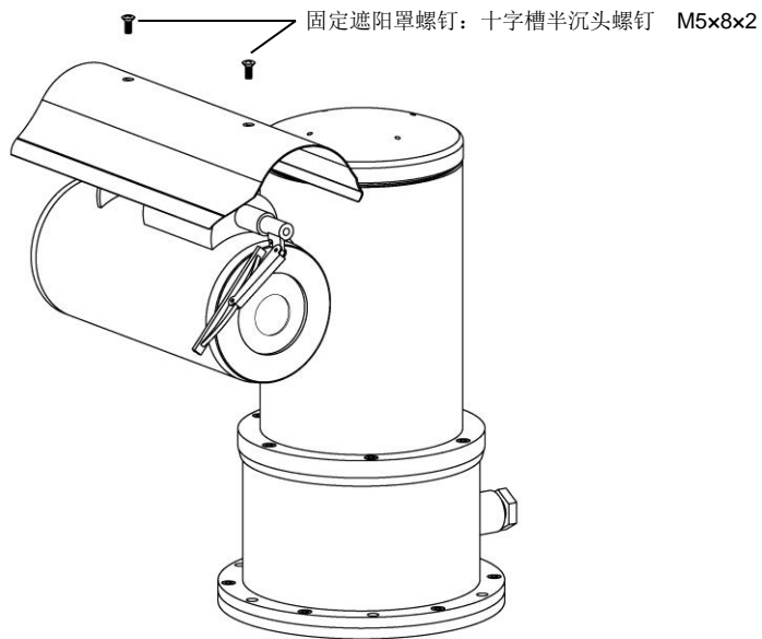
图 2.2.1.1 安装遮阳罩
