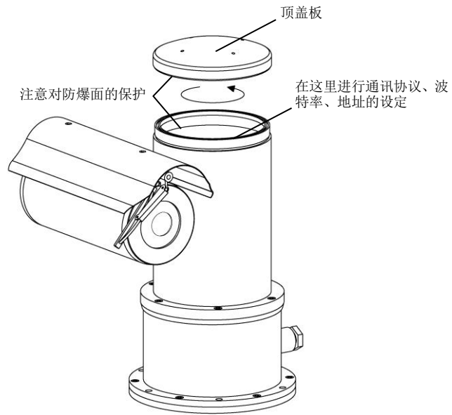
图 2.3.3.1 通讯设置
