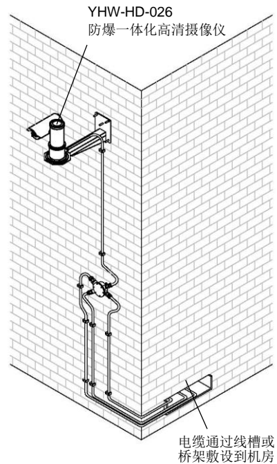
图 2.5.1.1 YHW-HD-026 支架安装
