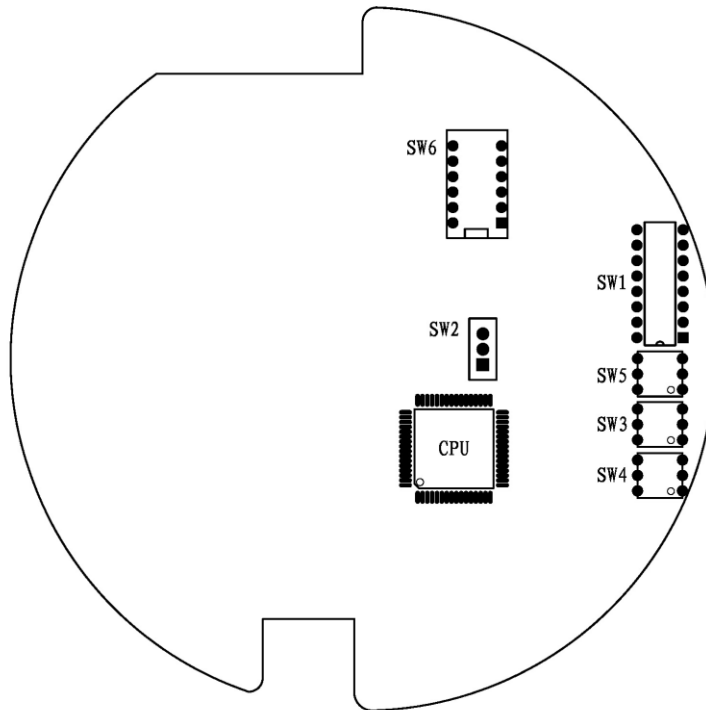
图 2.3.4.1. 主电路板外形图
