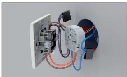
Obr. 1. RF Smart stmívač použitý v běžné instalaci
