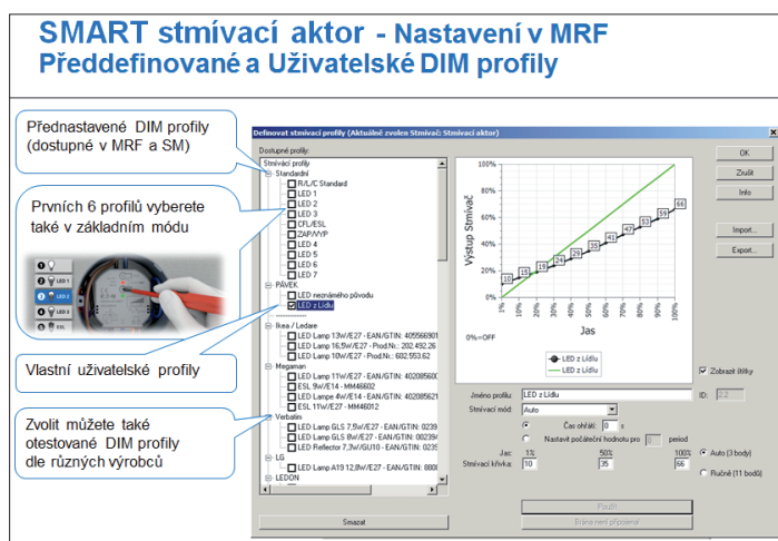
Obr. 2. Možnosti nastavení DIM profilů světelných zdrojů
