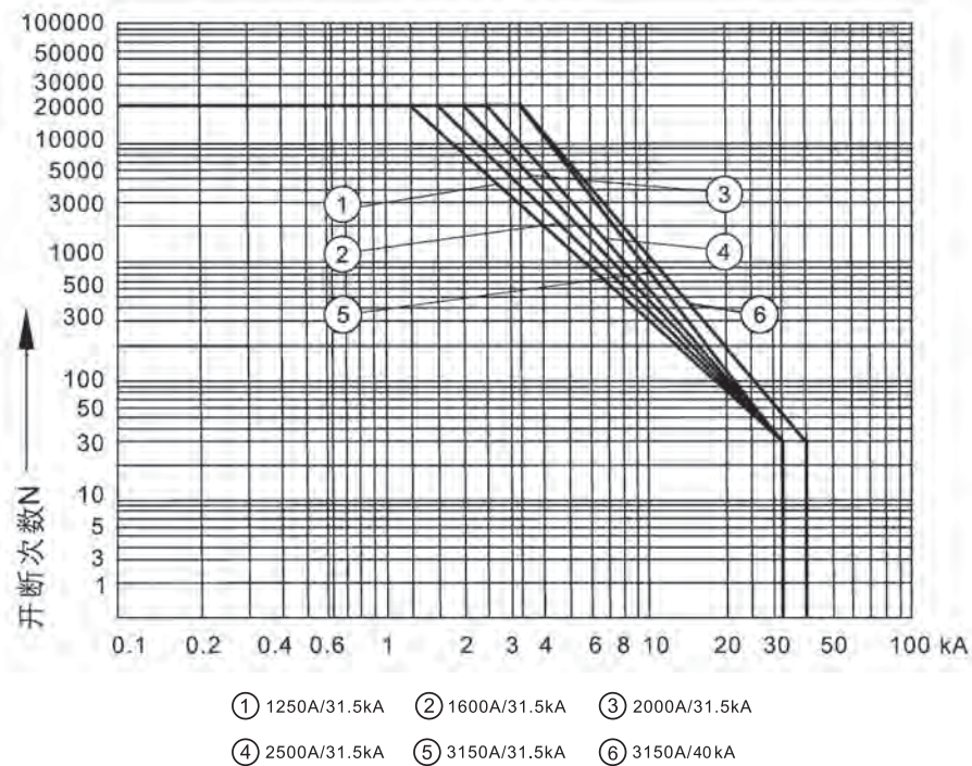
VN1-40.5E 真空灭弧室允许开断电流次数 N 与开断电流的关系
