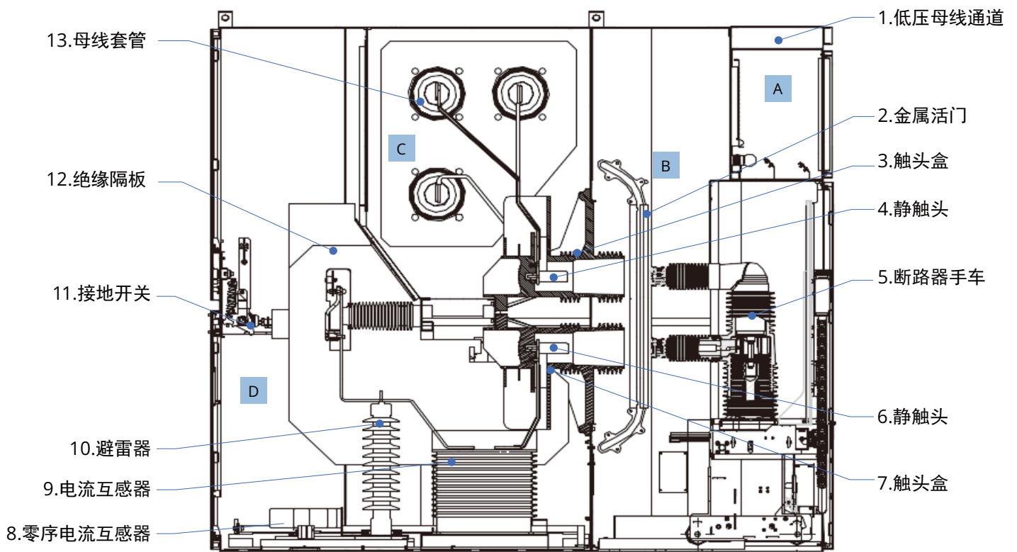
A—低压室 B—断路器室 C—母线室 D—电缆室
