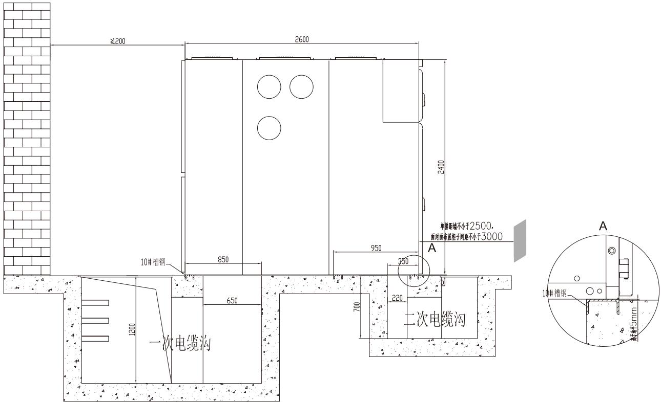
ET2 安装基础示意图
