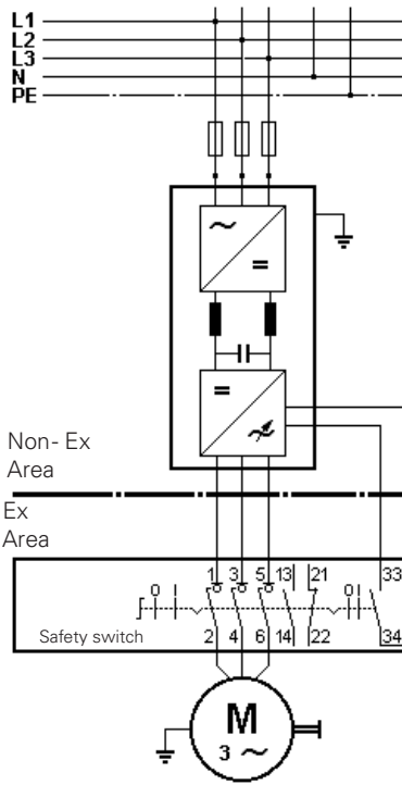
Wiring diagrams
