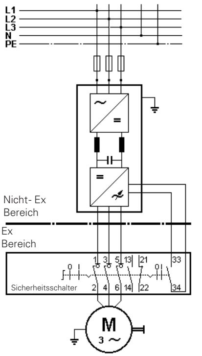
Anschlussbilder
