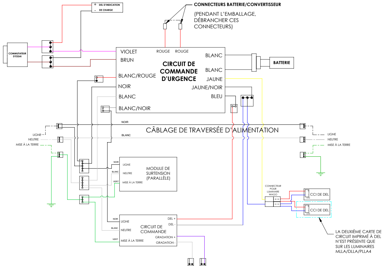
Figure 5. Schéma de câblage du système optionnel de protection contre les surtensions MLLA/DLLA/PLLA EM M2
