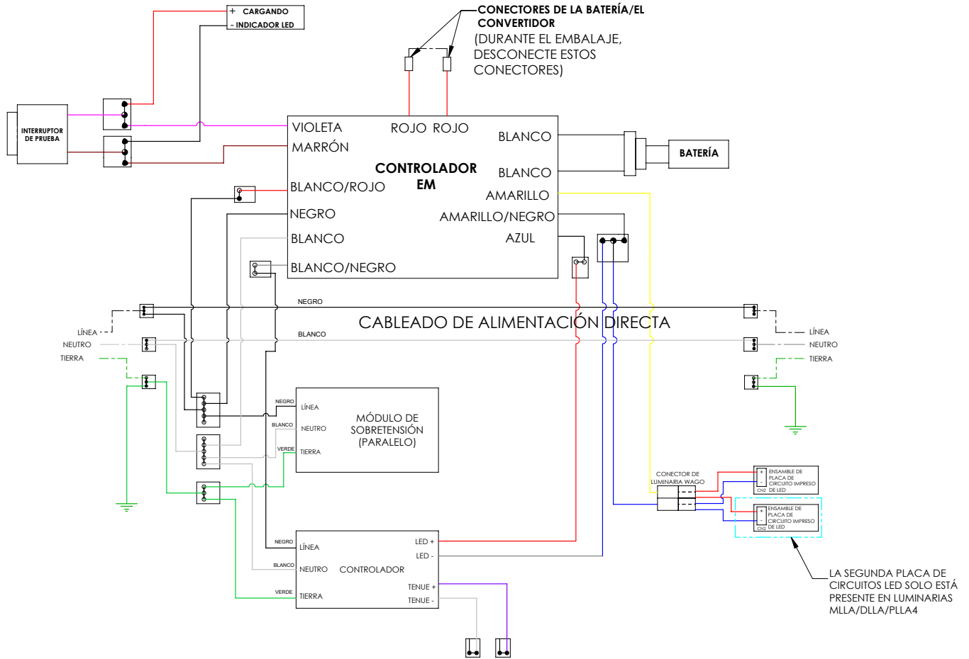
Figura 5: Diagrama de cableado del sistema de opción de sobretensión MLLA/DLLA/PLLA EM M2
