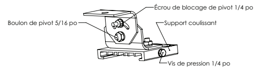
Figure 4. Détails du montage pivotant
