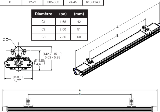
Figure 8 : TROUSSE Montage sur mât
