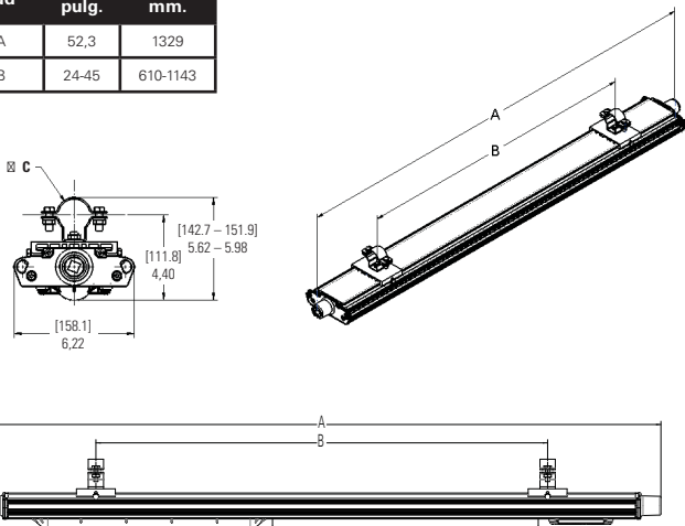
Imagen 8. KIT PM - Instalación del montaje en poste
