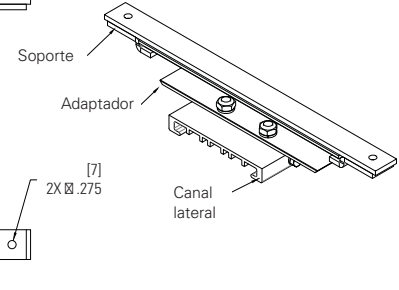
Imagen 7. Información del Kit de montaje MagnaPro Kit MP1054MTK
