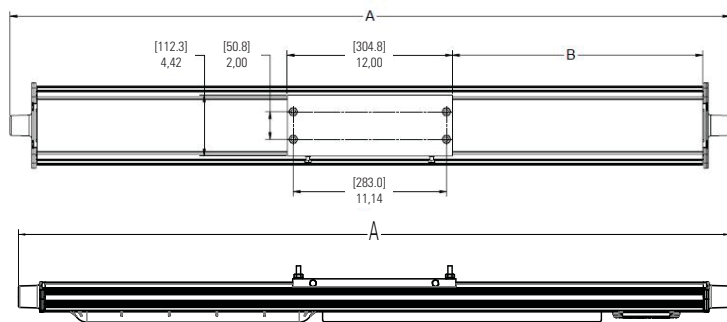
Imagen 3. Instalación del montaje trasero DP1057MTK
