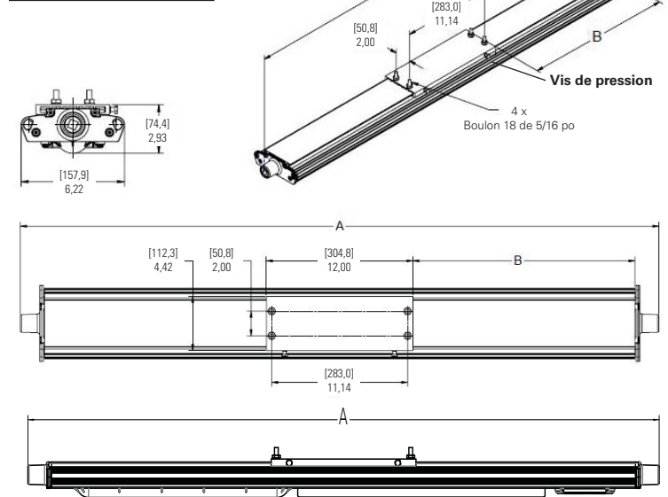
Figure 3. Montage arrière du DP1057MTK
