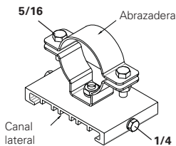
Imagen 9. KIT PM - Detalles del montaje en poste
