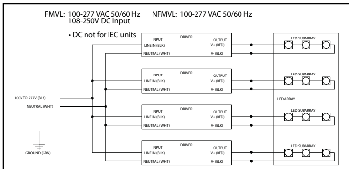
Figura 2 - Diagrama elétrico
