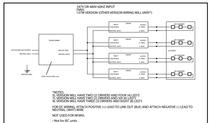
Figura 2 - Diagrama elétrico
