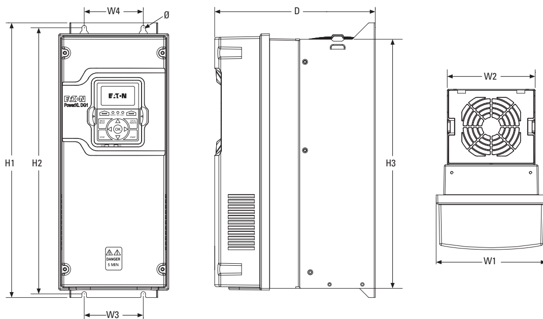
PowerXL 系列—DG1 尺寸图
