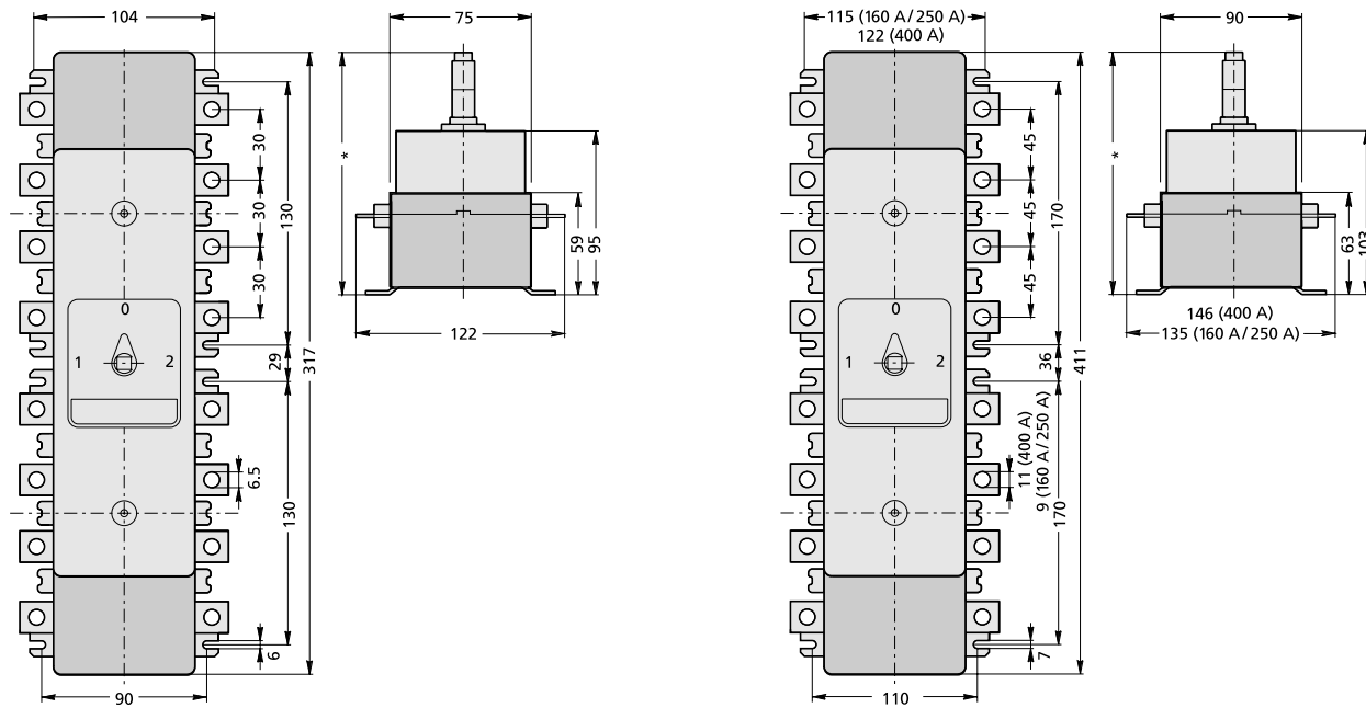
Перекидные выключатели Dumeco, тип DMV 160N.
