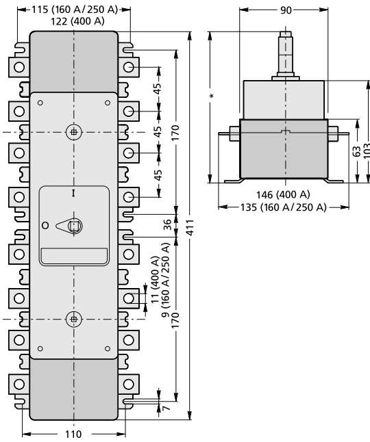
Многополюсные выключатели Dumeco, типы DMVS 160N, DMV 250N и DMV 400N.
