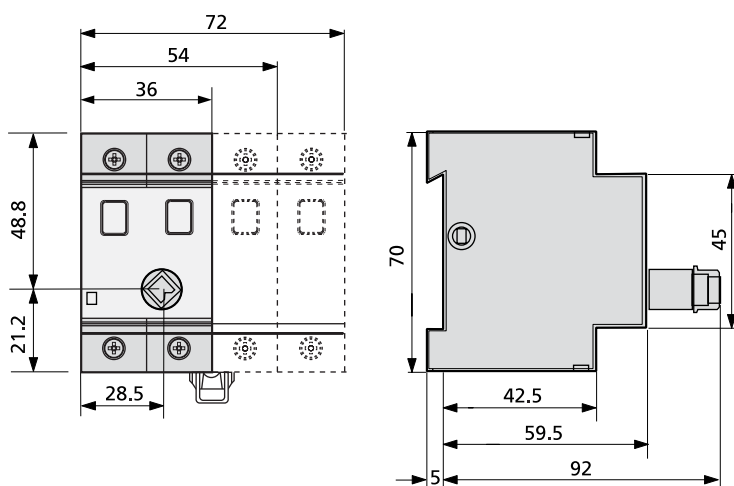
Disco, типы DMV 40 – DMV 63, без рукоятки.
