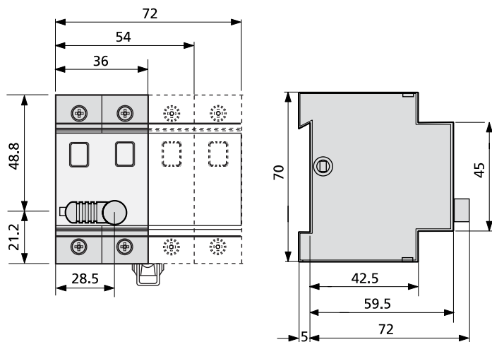
Disco, типы DMV 40 – DMV 63, с установленной рукояткой.
