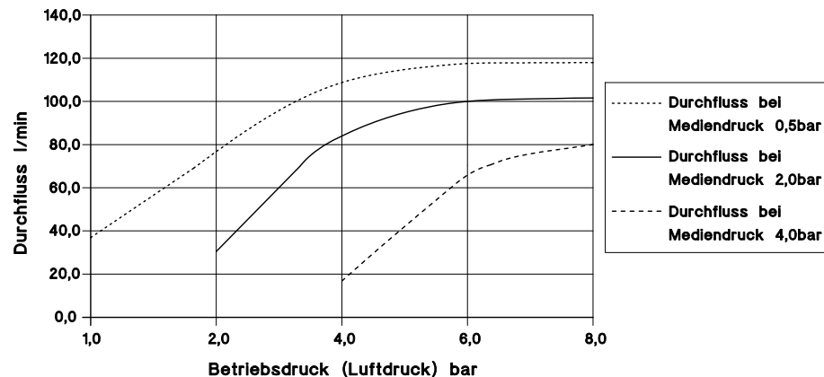
Durchflussskennlinie UMP40: Viskosität 30mm 2 /s
