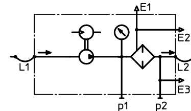
Filtereinheit ohne Verschmutzungsanzeiger
