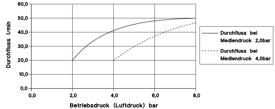
Durchflussskennlinie UMP40: Viskosität 1000mm 2 /s
