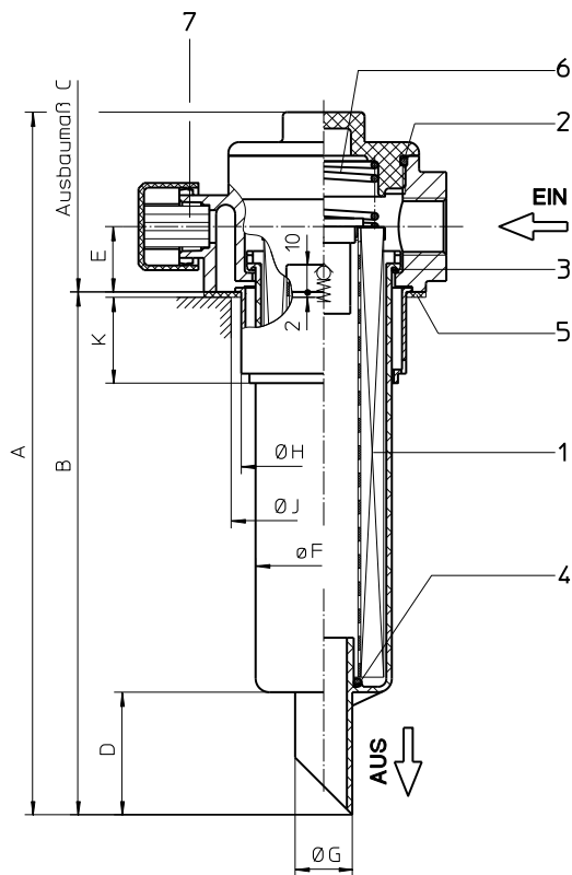
Ansichten TEFB 55, 70
