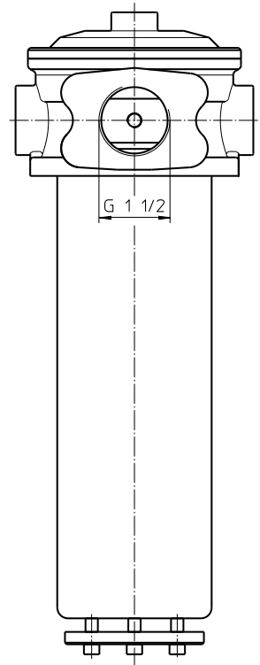
Ansicht X Ausführung G 1 1/2"
