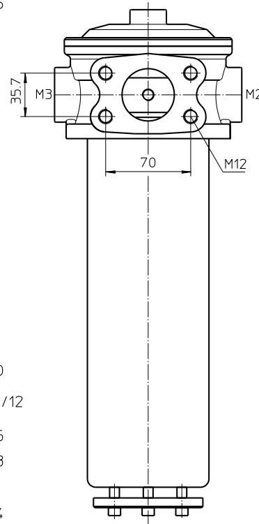
Ansicht X Ausführung SAE 1 1/2"
