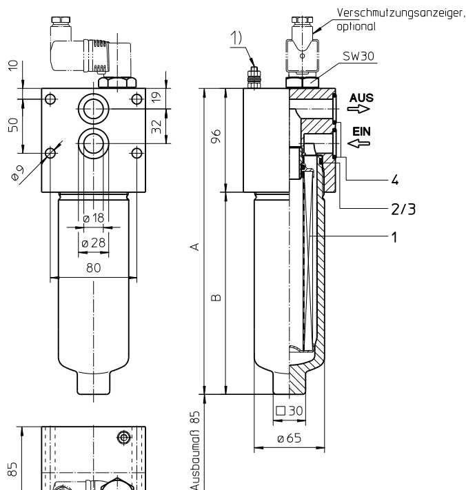
Ausführung HPF 60-150
