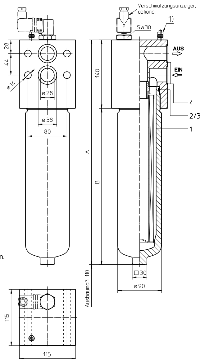
Ausführung HPF 170-450
