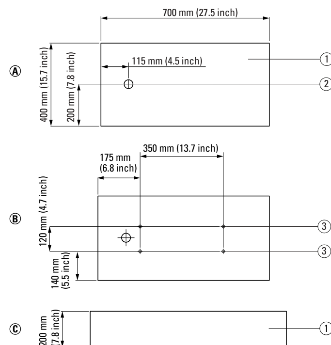
Figure 2. Green Motion DC 22 Unter-, Ober- und Vorderansicht des Betonsockels für die EV-Ladesäule mit Abmessungen
