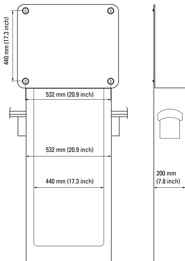
Figure 1. Vorder- und Seitenansicht der Green Motion DC 22 Ladesäule mit Abmessungen in mm
