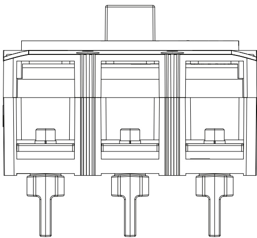
PDG4X3T800RC
