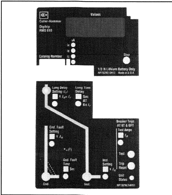
Fig. 3.4 Digitrip RMS 610 Type LIG
