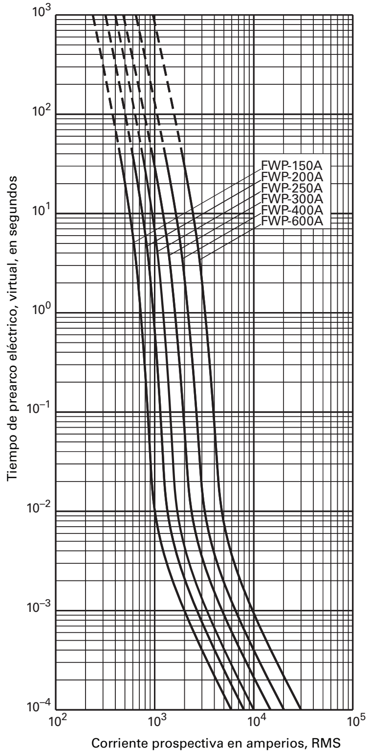
Curvas características de corriente-tiempo. Fusión mínima
