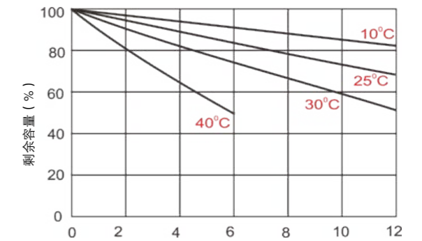
自放电特性
