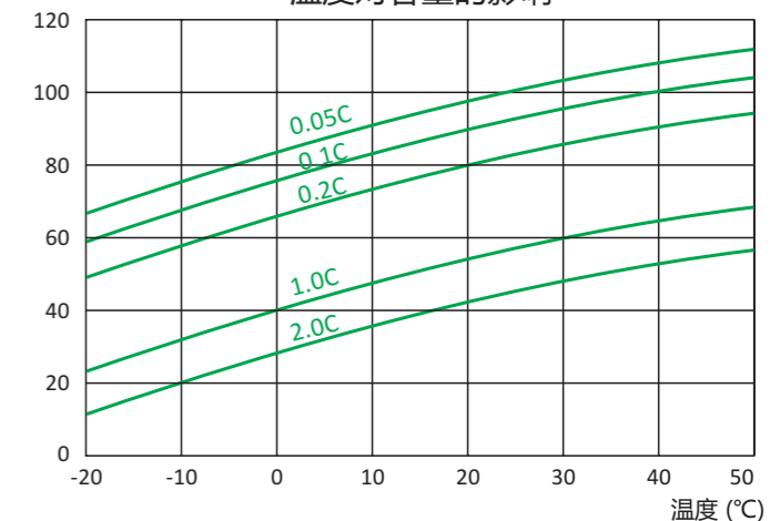
温度对容量的影响
