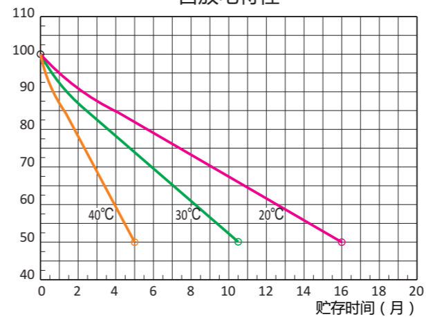
自放电特性
