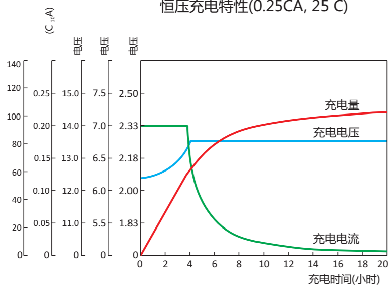
恒压充电特性(0.25CA, 25°C)
