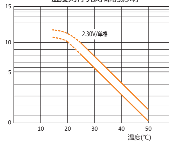
温度对浮充寿命的影响
