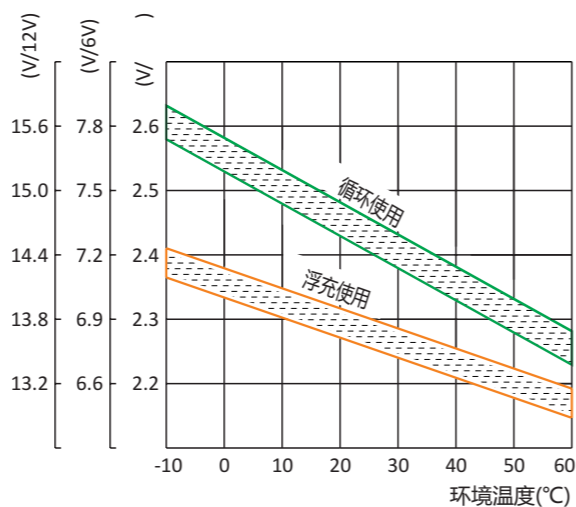
充电电压与温度的关系
