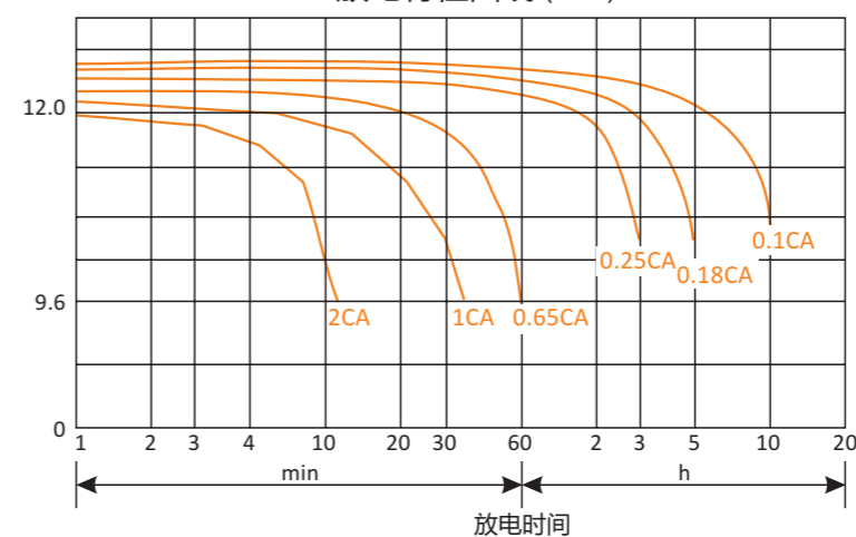
放电特性曲线 (25°C)
