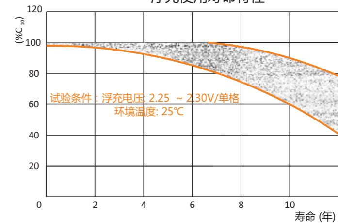
浮充使用寿命特性
