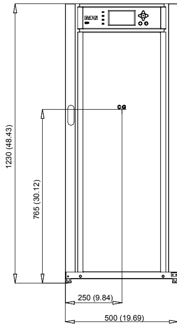
前视图
