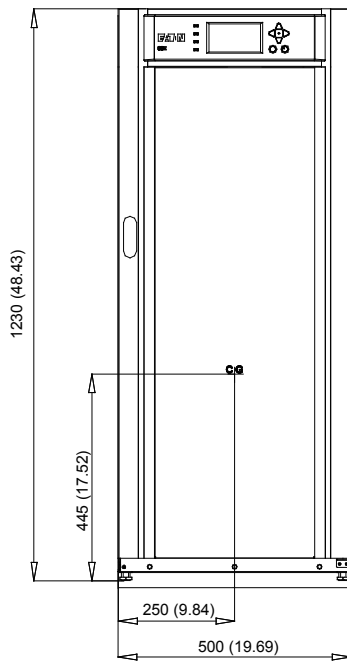
前视图
