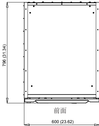
俯视图
