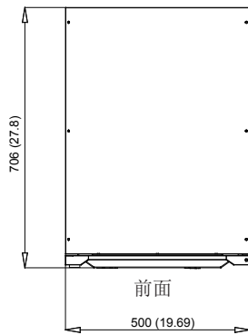
俯视图
