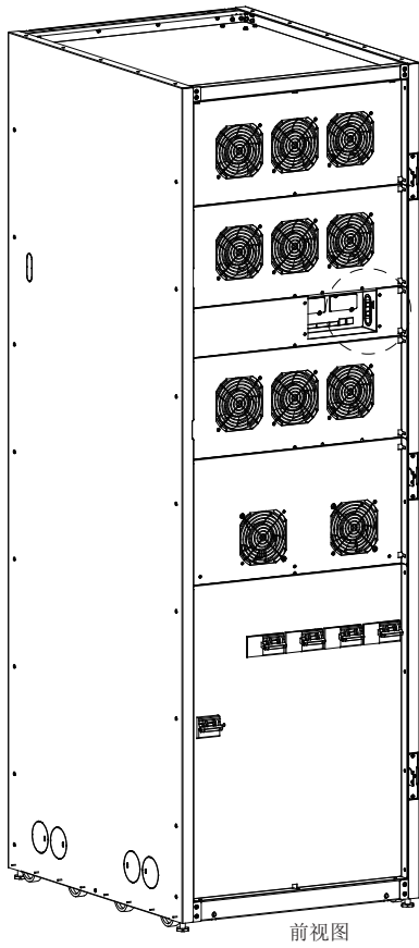
93E 60-80 kVA
