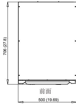
俯视图
