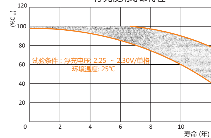
浮充使用寿命特性
