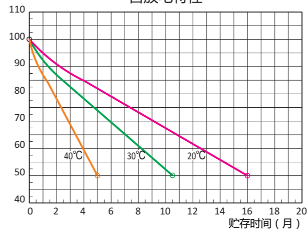
自放电特性
