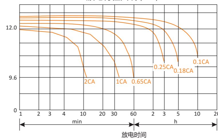
放电特性曲线 (25°C)
