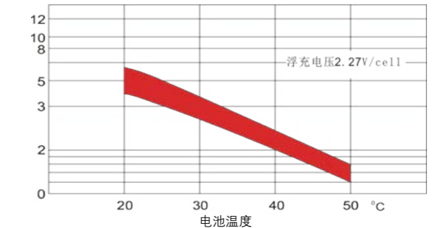
ETNHW12-9Ah/20Ah 温度对浮充寿命影响
