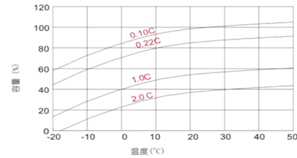
温度对容量影响
