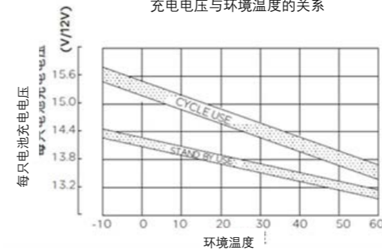
充电电压与环境温度的关系
