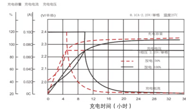
充电特性曲线
