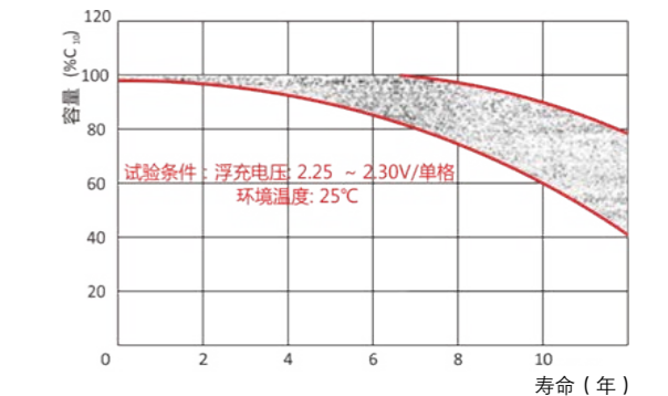
浮充使用寿命特性
