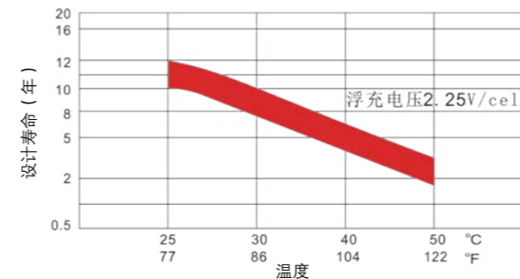
ETNHW12-38Ah~ETNHW12-250Ah 温度对浮充寿命影响
