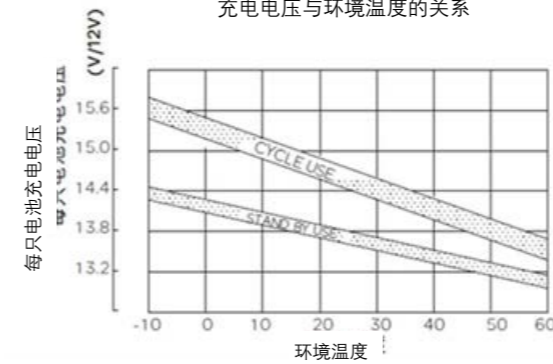
充电电压与环境温度的关系
