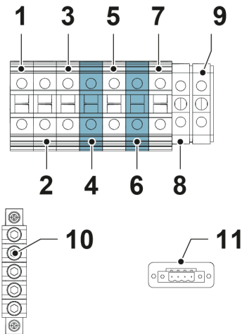
Figura 11. Terminali del cavo di alimentazione dell'UPS per unità monofase
