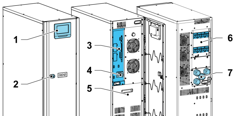
Figura 2. Panoramica interna del telaio standard per l'UPS Eaton 91PS/93PS 8-10 kW
