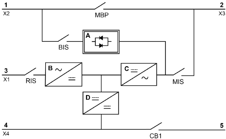
Figura 7. Schema di cablaggio dell'UPS comprensivo di soluzione MBS
