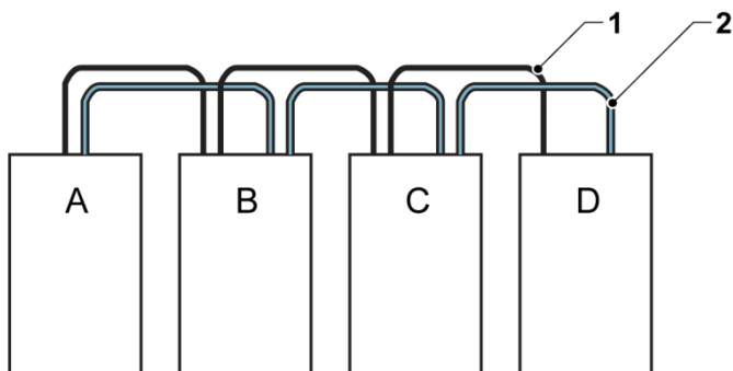
Figura 19. Cablaggi CAN semplificati e pull-chain per sistemi UPS paralleli
