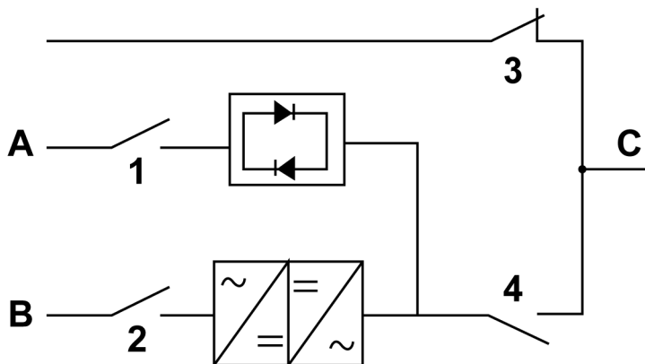
Figura 33. Modalità di bypass per manutenzione
