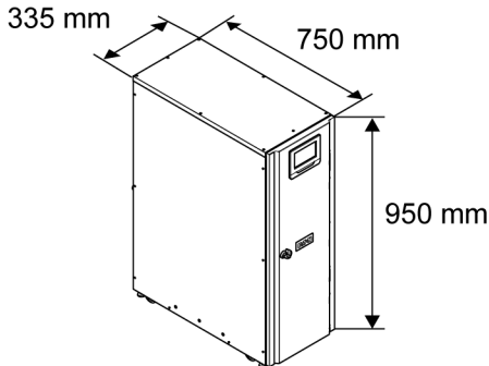
Figura 9. Dimensioni dell'UPS Eaton 91PS/93PS 8-10 kW
