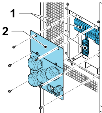
Figura 12. Ubicazione della piastra passacavi e dei connettori
