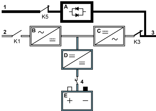
Figura 4. Percorso della corrente attraverso il sistema UPS in modalità Energy Saver System (sistema a risparmio energetico)
