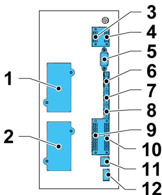
Figura 22. Interfacce di comunicazione sul telaio dell'UPS 91PS/93PS 8-10 kW
