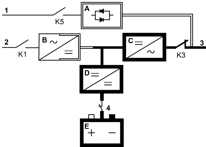
Figura 5. Percorso della corrente attraverso il sistema UPS in modalità batteria
