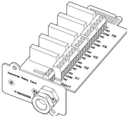
Figura 17. Scheda relè industriale INDRELAY-MS
