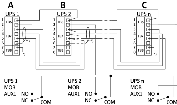
Figura 20. Cablaggi CAN semplificati e pull-chain per sistemi UPS paralleli dotati di interruttori MOB
