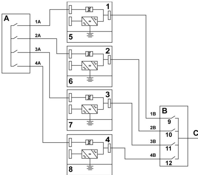
Figura 18. Principio dei sistemi UPS in parallelo
