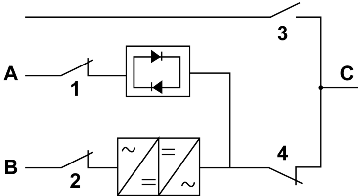
Figura 32. Posizioni normali degli interruttori
