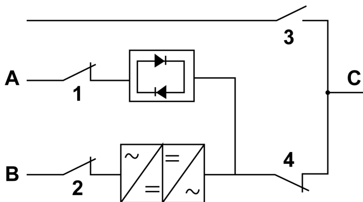
Figura 35. Posizioni normali degli interruttori
