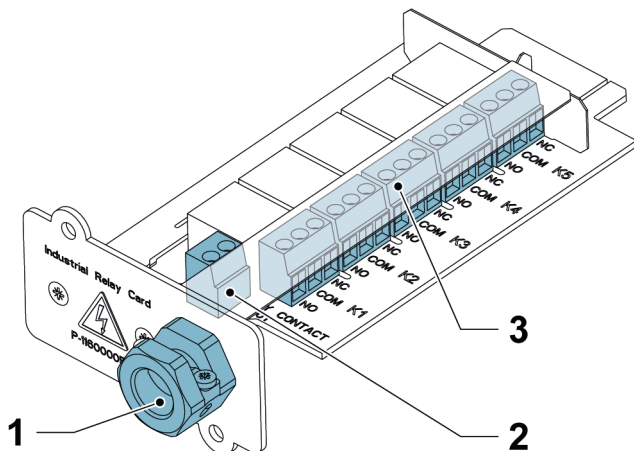
Figura 30. Relè
