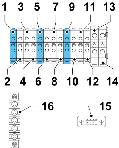
Figura 10. Terminali del cavo di alimentazione dell'UPS per unità trifase
