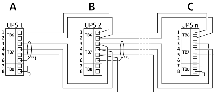
Figura 21. Cablaggi CAN semplificato e pull-chain per sistemi UPS paralleli privi di interruttori MOB
