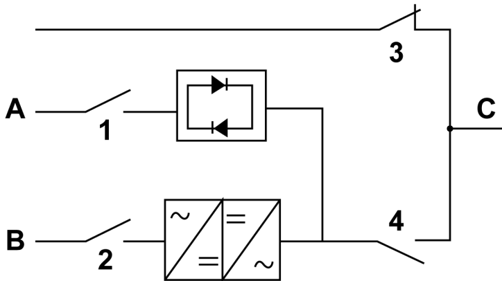
Figura 34. Modalità di bypass per manutenzione
