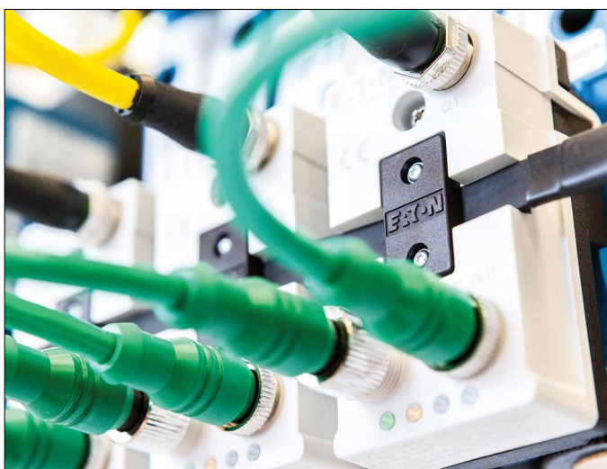
SmartWire-DT anche fuori dal quadro elettrico. Consente l'individuazione degli errori in modo più semplice e immediato.
